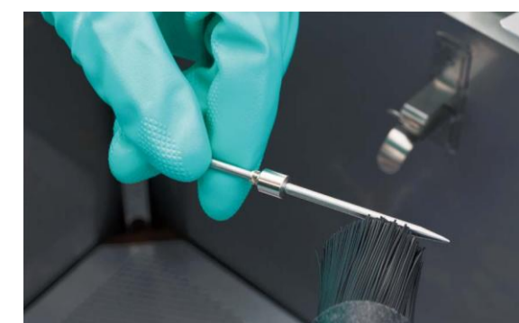
图22 清洗枪针
